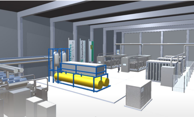
Rendering des sich im Aufbau befindlichen Hydrogen Lab Görlitz auf dem Gelände des Siemens Energy Campus
